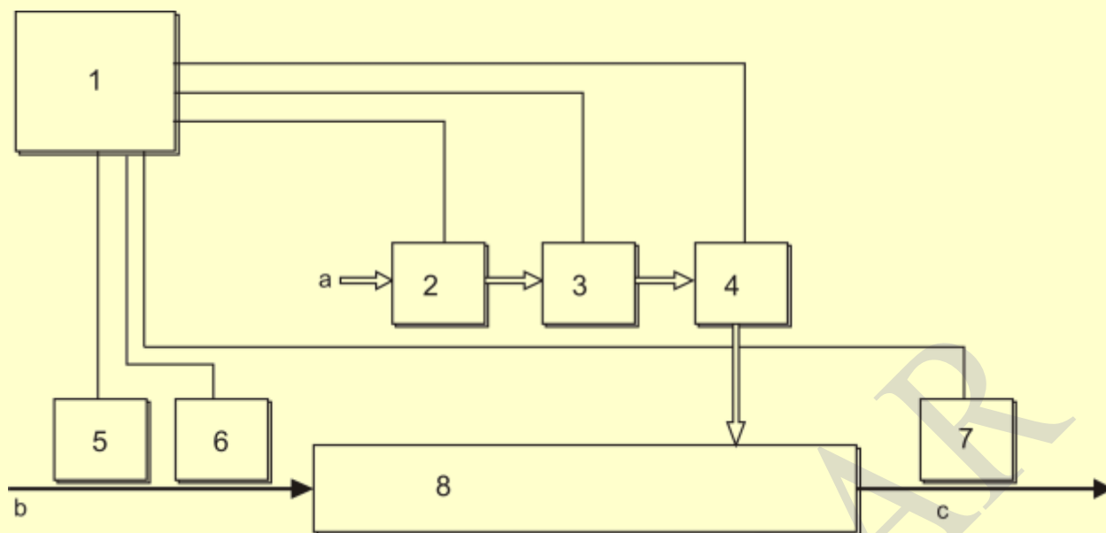
Рис. 5.1. Структурная схема системы доувлажнения «МИКРОРАДАР-200-02».
