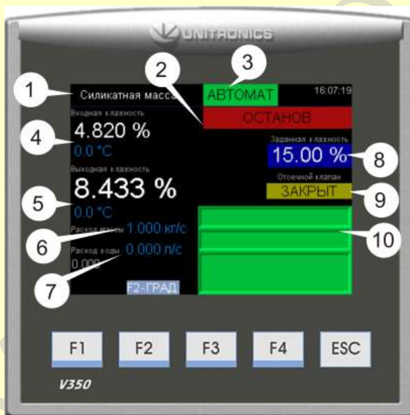
Рис. 5.1.1. Экран ПЛК в режиме «Автомат»
