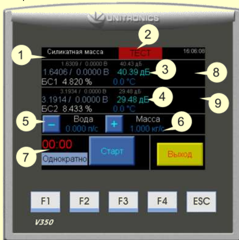
Рис. 5.3.1. Экран ПЛК в режиме «Тест»
