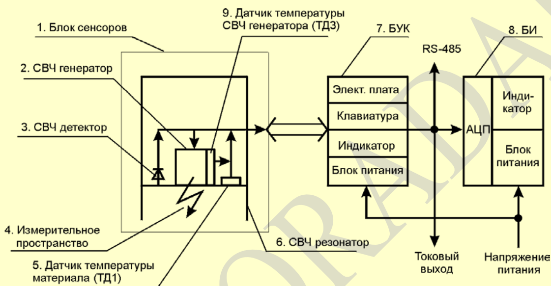
Рис. 6.1. Функциональная схема влагомеров «Микрорадар-114А(Д)13К» и «Микрорадар-114А(Д)13В»
